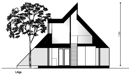
Lõige
