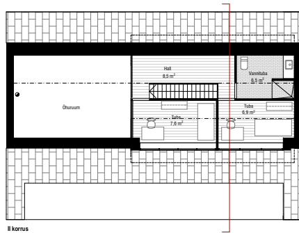
II korrus
